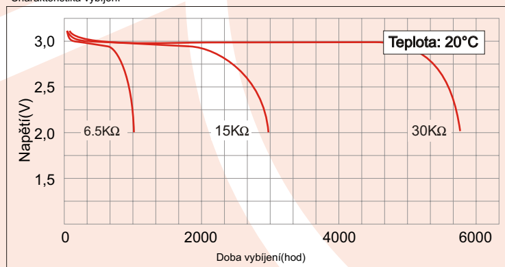
Charakteristika vybíjení
