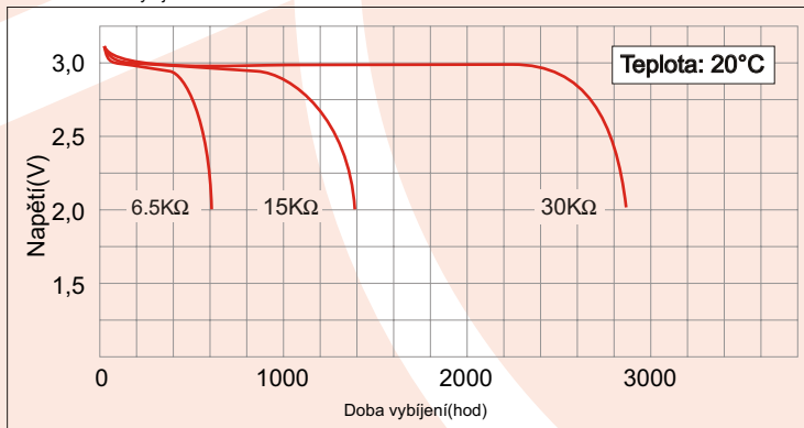
Charakteristika vybíjení
