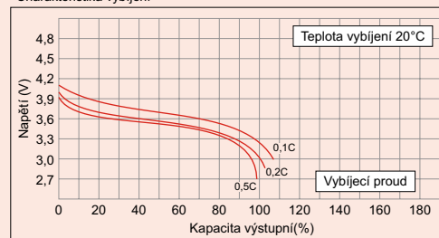
Charakteristika vybíjení
