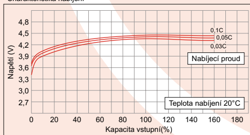
Charakteristika nabíjení
