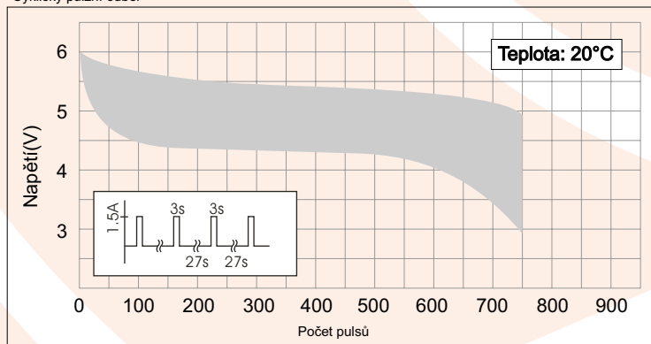
Cyklický pulzní odběr
