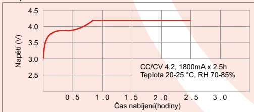
Nabíjecí charakteristika
