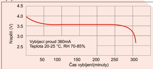
Vybíjecí charakteristika
