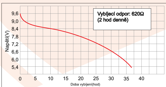
Charakteristika vybití
