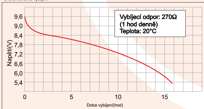
Charakteristika vybití
